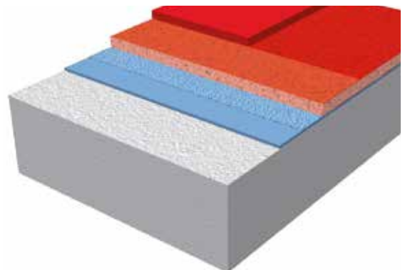
Mit Einstreuchips
