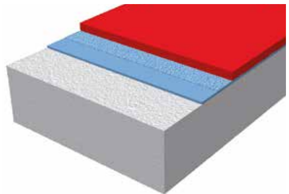
Glatte Verlaufsbeschichtung
